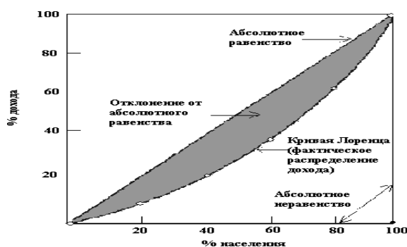
Рисунок 12.1. - Кривая Лоренца
